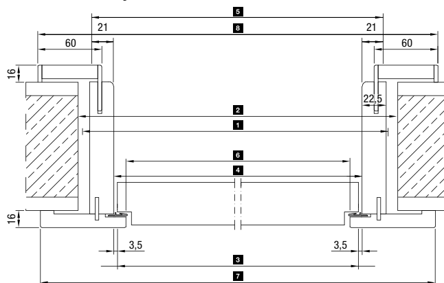
Vodorovné řezy
