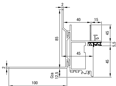
Kótování zárubně Zeroline
